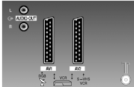
Salida de enchufes L-R AUDIO OUT 2 cables de audio RCA
